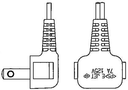
電源プラグ (ショートコード仕様)
