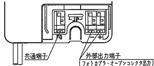
外部出力端子部 (端子カバー解放時)
