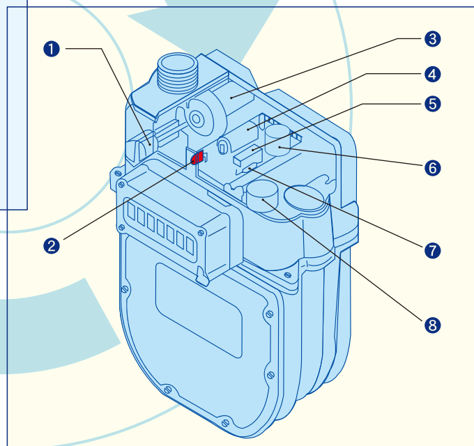
構造図
