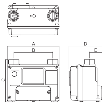
型式 EK25BL、EK4BL
