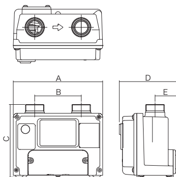
型式 EK25NL、EK4NL
