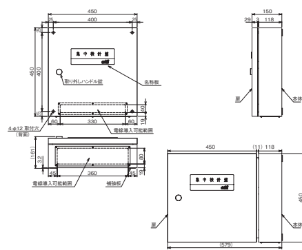
型式 KILVIS-HA (屋内仕様)
