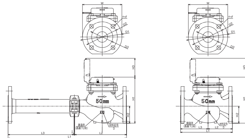
型式 GFDW50～100mm
