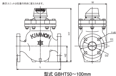
型式 GBHT50~100mm
