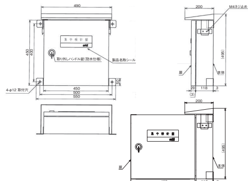
型式 KILVIS-HA (屋外仕様)
