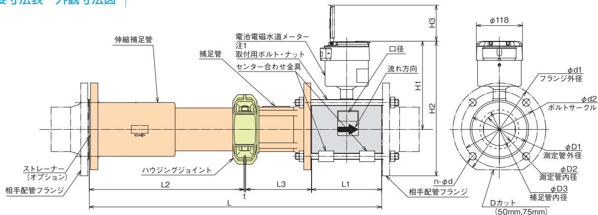
主要寸法表・外観寸法図
