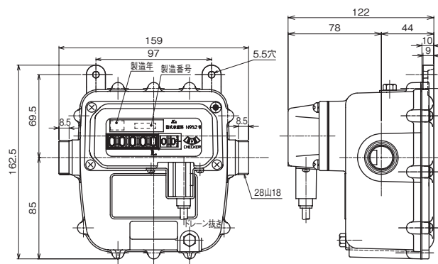
型式 GNDR-6
