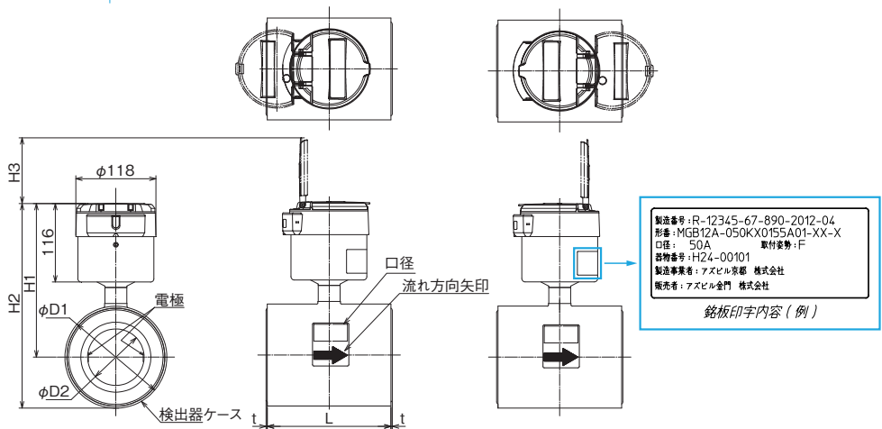
主要寸法表・外観寸法図
