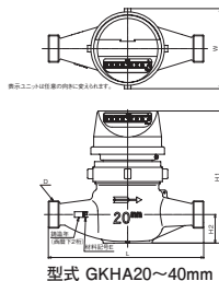
型式 GKHA20~40mm
