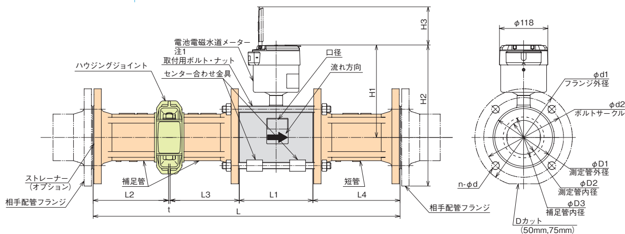
主要寸法表・外観寸法図
