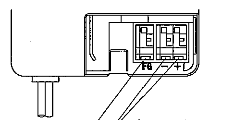
外部出力端子部 (端子カバー開放時)
